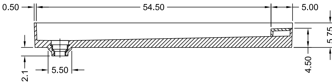
SECTION A-A
